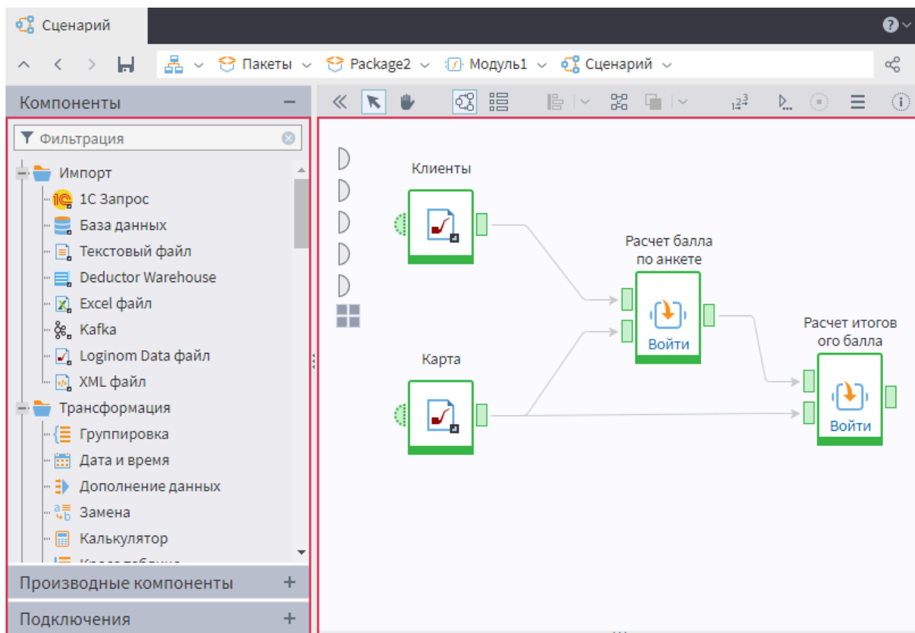
Рисунок 1. Страница «Сценарий»
